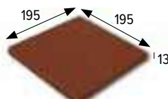
Remate 20/RE20 Edge 20 195x195x13 mm
